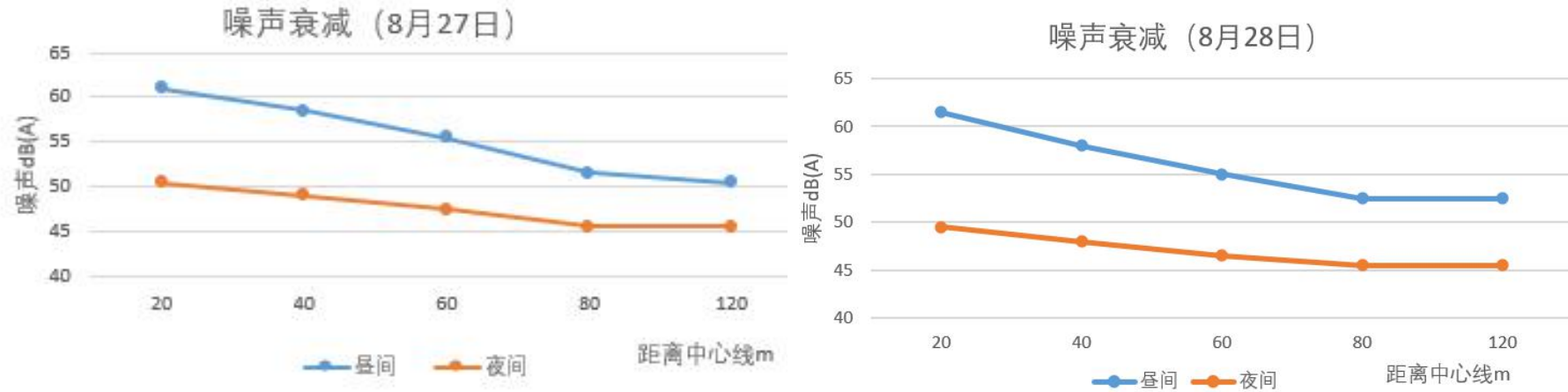
图 7.3-2 断面处昼间和夜间噪声衰减曲线
