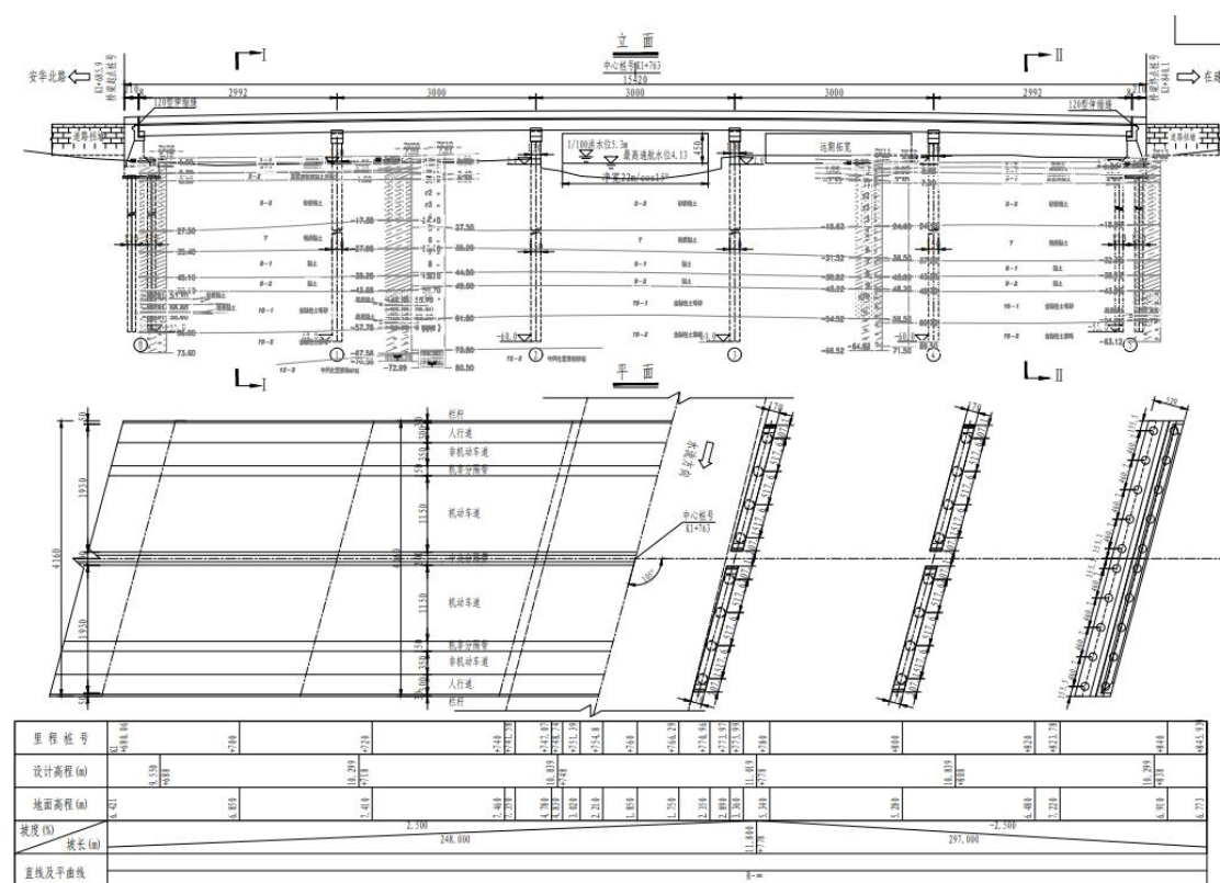
图 8.2-4 朝阳河大桥立面图
